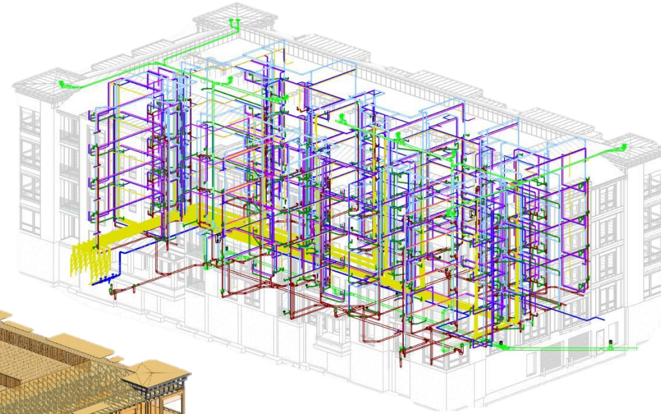
MEP Modelling
